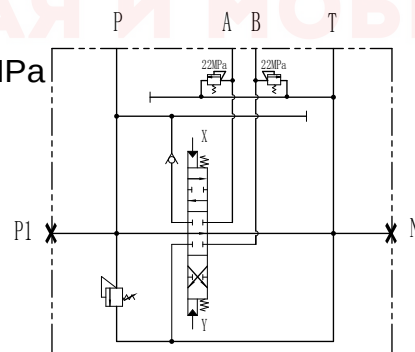
液压原理图
