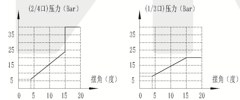
输出压力特性曲线
