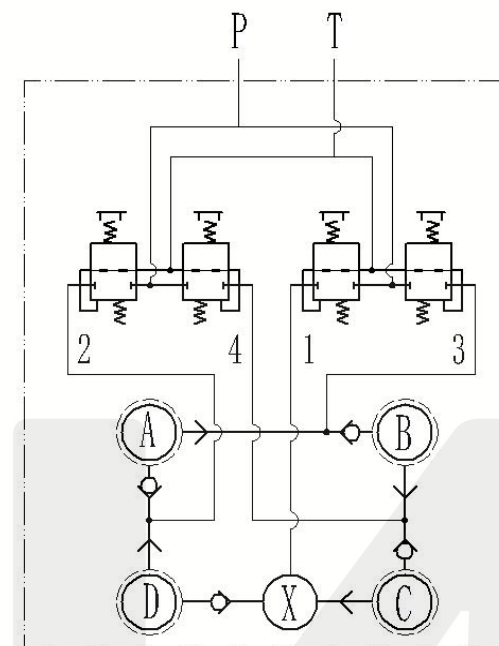
液压原理图
